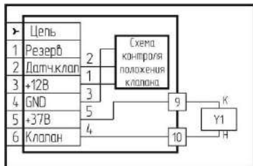
Рисунок 4 – Клапан КЗЭУГ. Схема электрическая принципиальная.
